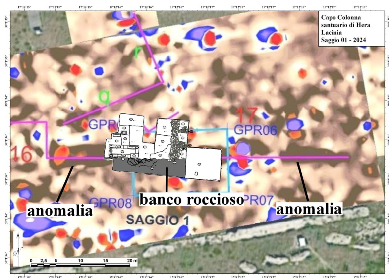
Fig. 15. Anomalia lineare individuata con le indagini geonostiche e rapporto con il banco roccioso individuato nello scavo (restituzione M. Silani).
